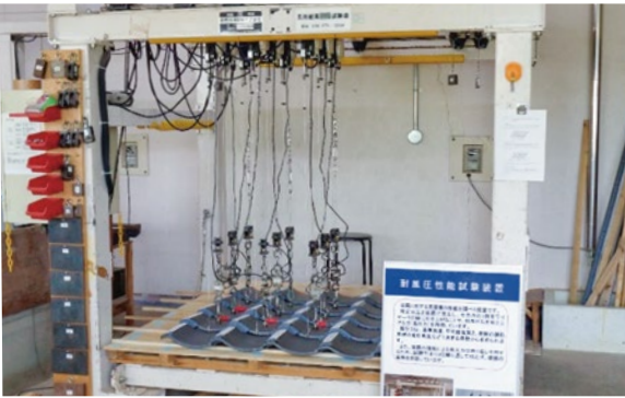
瓦風圧試験の様様
