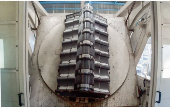
耐震試験の様様
